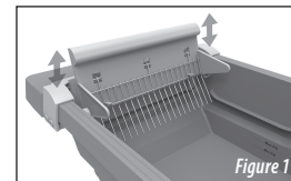
Rake assembly
