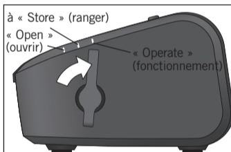
Fermer et tourner le loquet de verrouillage facile en position « Operate » (fonctionnement)
